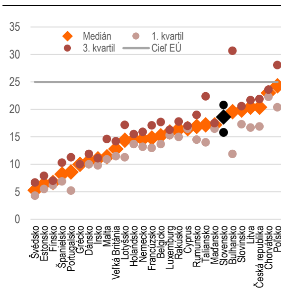
Graf 21: Ročná priemerná koncentrácia PM 2,5
